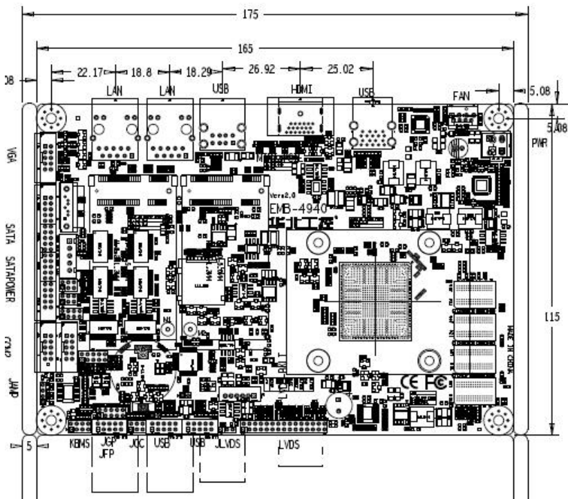
EMB-4940 V2.0 接口位置和尺寸图
